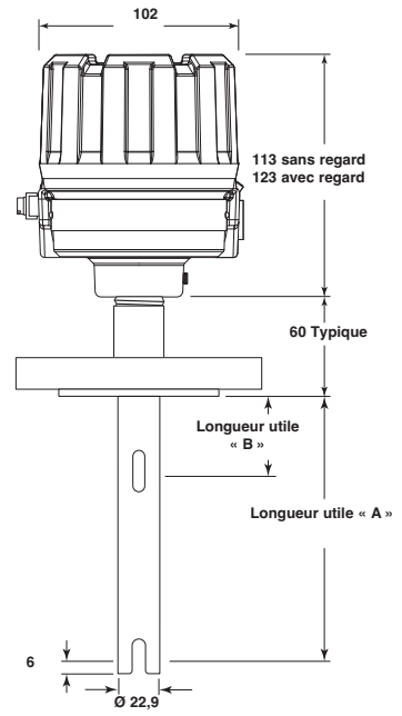
962 - Raccordement à bride
