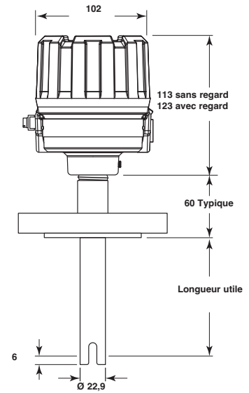
961 - Raccordement à bride
