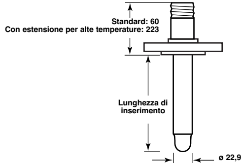
Sensore flangiato
