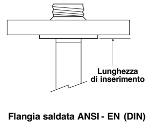
Flangia saldata ANSI - EN (DIN)
