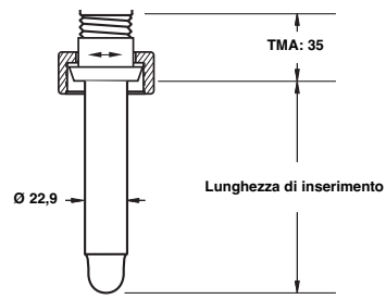
DIN 11851
