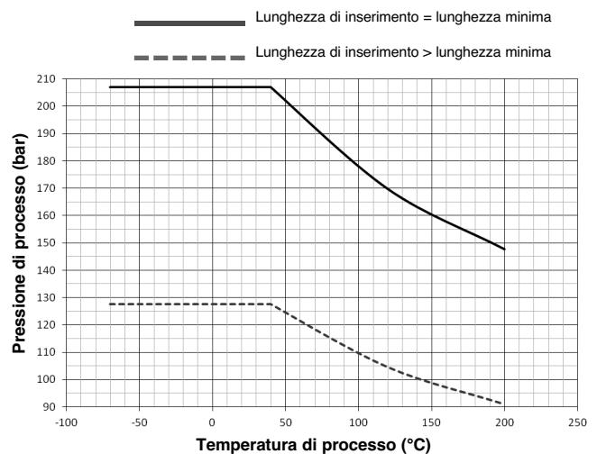
Sensori TMC/TMD con codice materiale A o D
