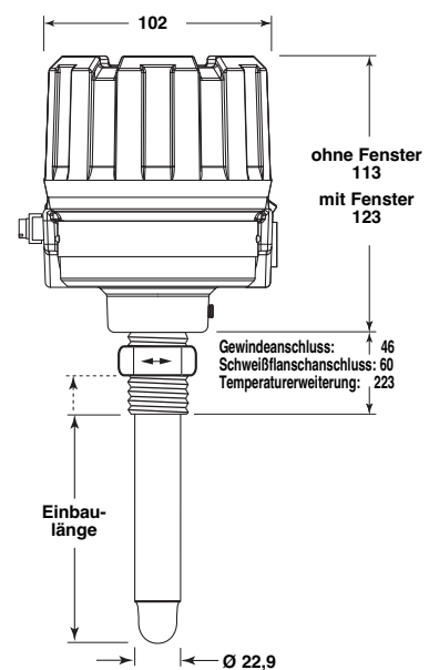
Modell TD2 mit Kompaktversion und TMA/TMB-CIP-Sensor
