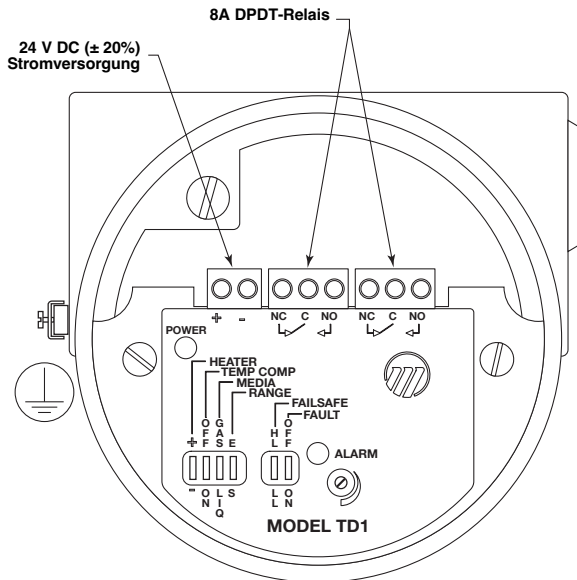
Verdrahtung TD1
