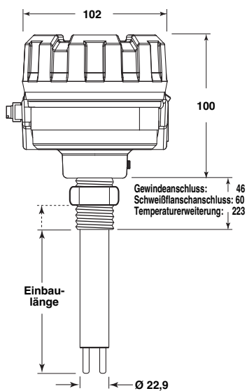
Modell TD1 mit TMC/TMD-Standardsensor
