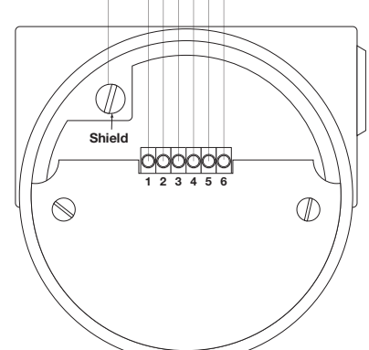
TD2 Getrenntversion-Sensoranschlüsse
