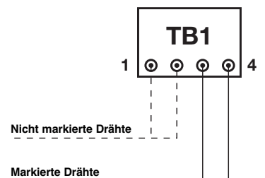
TD2 Getrenntversion-Sensoranschlüsse
