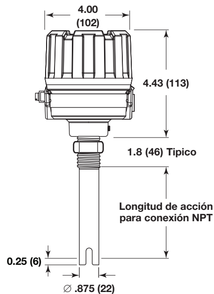
Modelo 961 con cubierta de aluminio moldeado con conexión NPT
