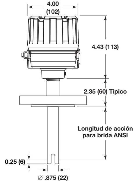
Modelo 961 con cubierta de acero inoxidable moldeado y brida ASME
