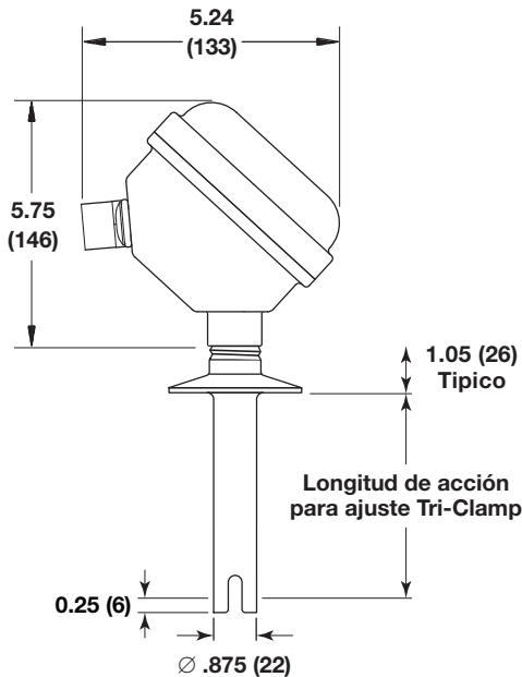
Modelo 961 con cubierta higiénica con relleno Tri-Clamp® 16 AMP
